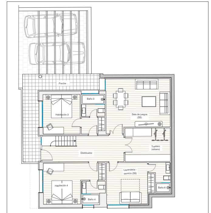
PLANTA BAJA
