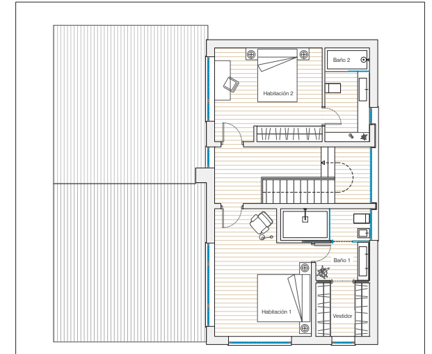
PLANTA SEGUNDA
