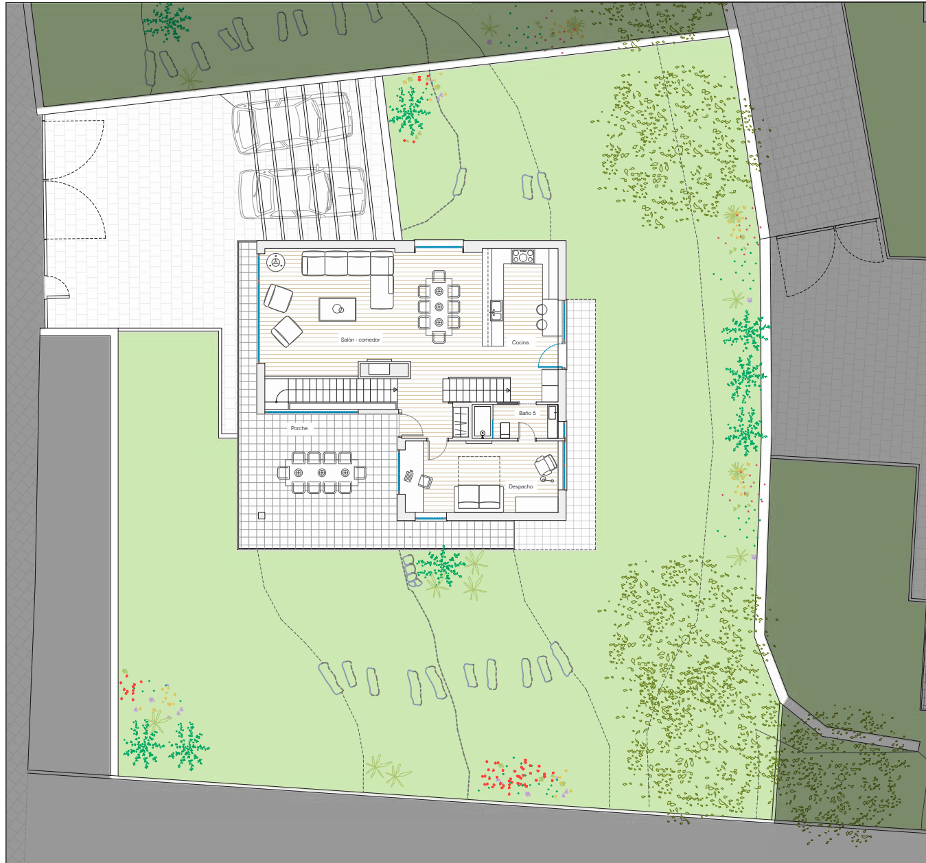
PLANTA PRIMERA
